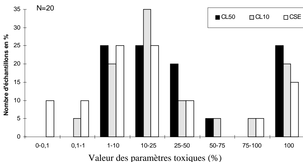
Figure 38 : Répartition des réponses de l'essai hydre ( CL_{50} , CL_{10} et CSE) à 96h sur N=20 échantillons d'eaux interstitielles.
