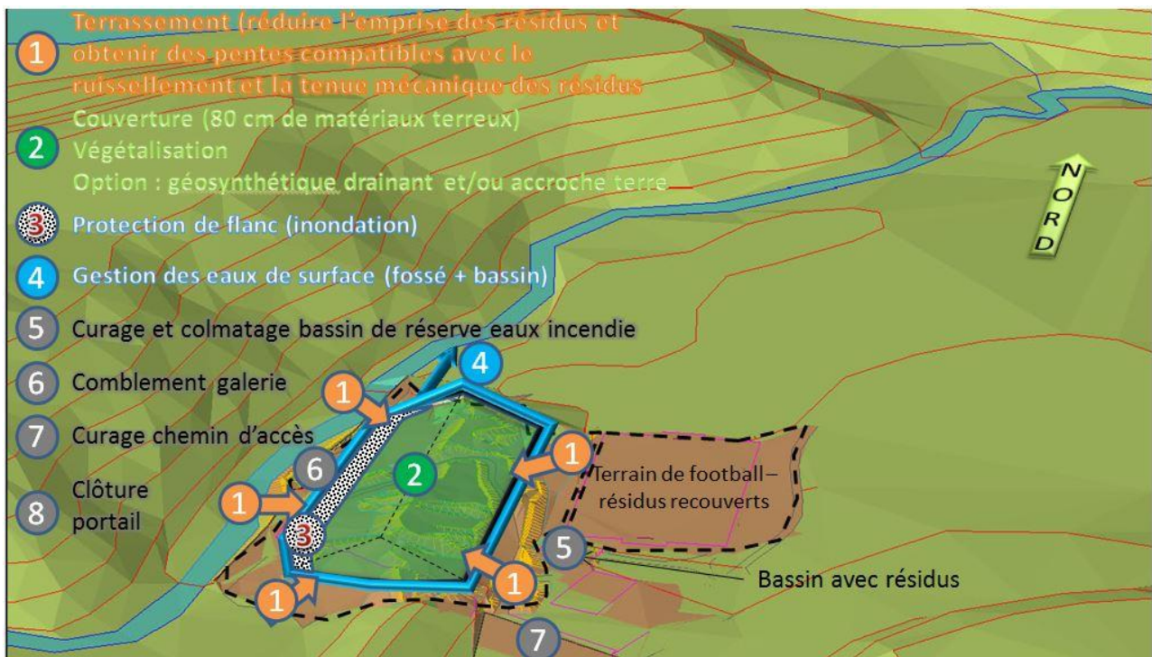
Figure 4. Schéma conceptuel du réaménagement du site des Fonderies.
